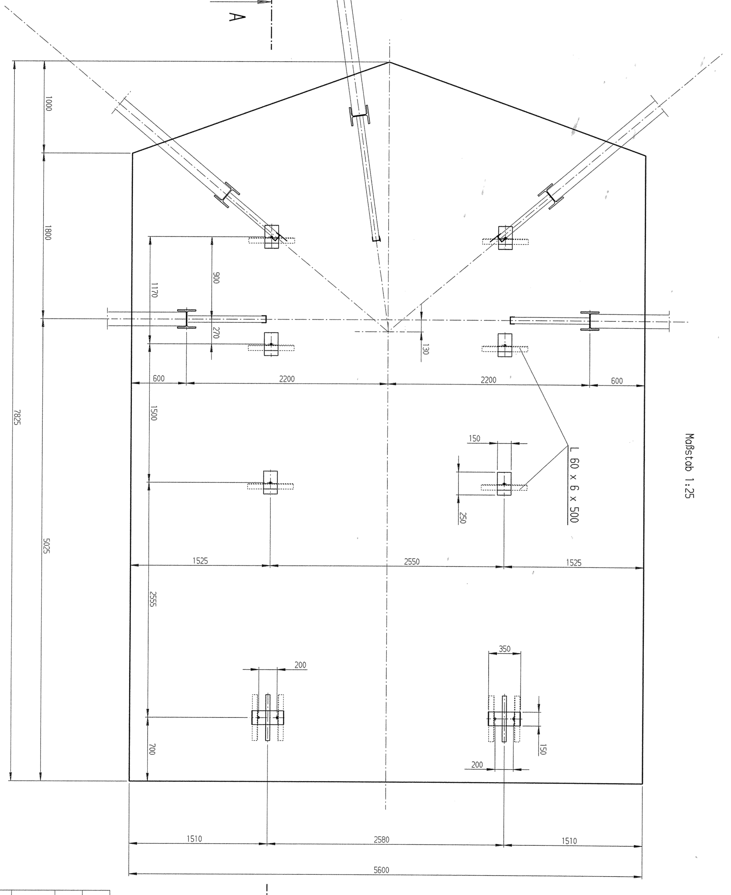
Kolbertisch 1:25
